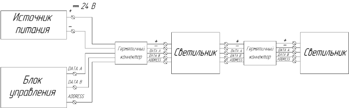
Рис.2. Схема подключения светильника
