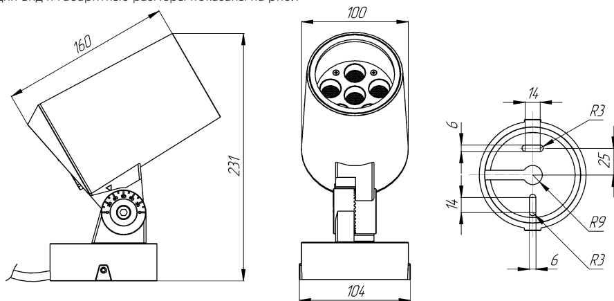
Рис.1. Габаритные размеры
