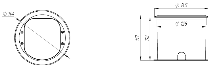
Рис.1. Габаритные размеры
