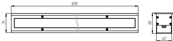
Рис.1. Габаритные размеры
